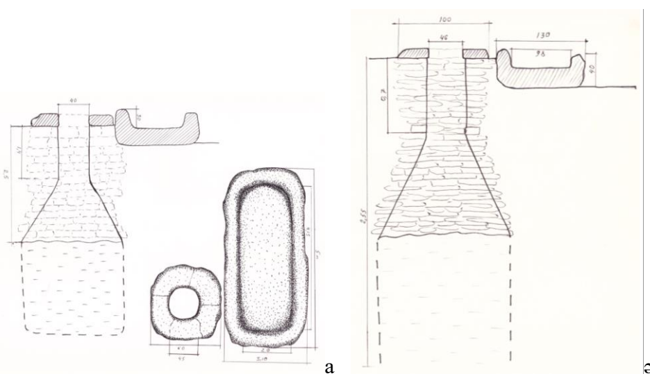
9-сур. Тұщыайрық құдықтарының сызбасы: а) №3 құдық, кескінді сызбасы; ә) №4 құдық, әуіт және тас ас.
