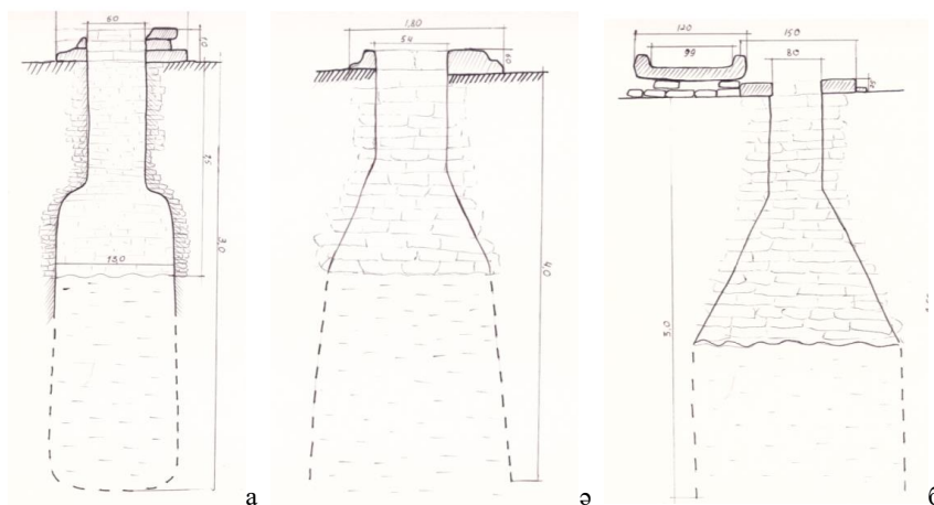
5-сур. Ащыайрық құдықтарының сызбасы: а) No1-құдықтың кескінді сызбасы;
